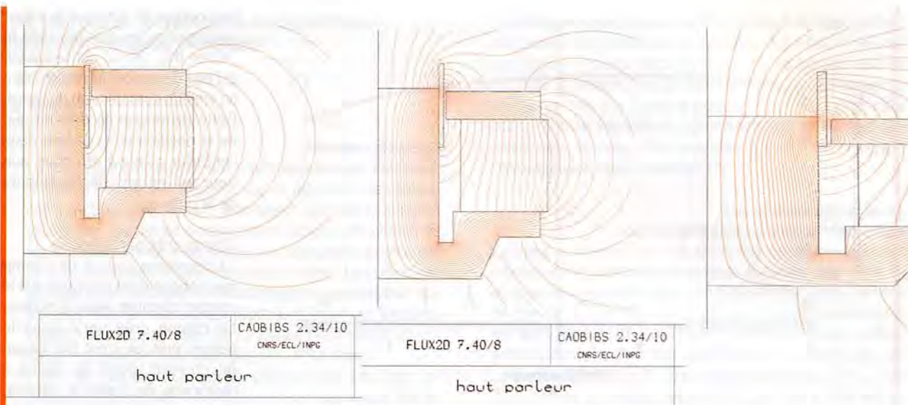
(a) Bobine basse
