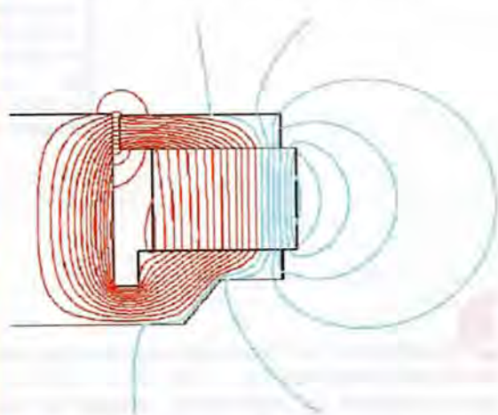
Fig. 2 : Lignes de champ créées par l'aimant dans le moteur
