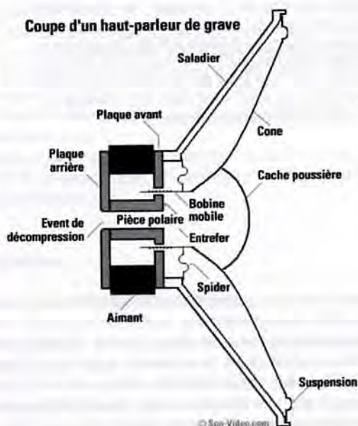
Fig.1 : Structure classique de haut-parleur électrodynamique
